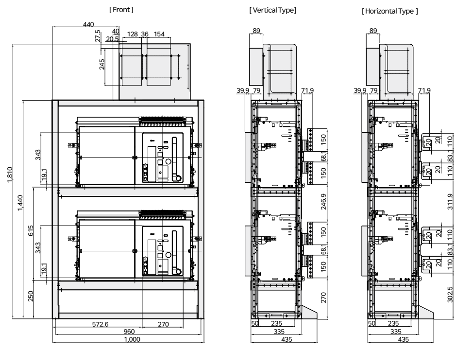
HGN50 ~ 63 D, 3P
